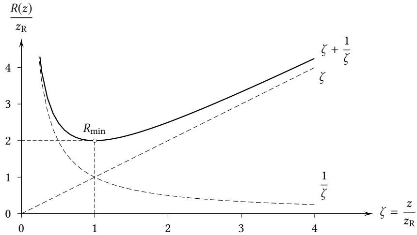
Abb. 2: Normierte Abhängigkeit des Krümmungsradius der Phasenfronten vom Abstand von der Strahltaile.
